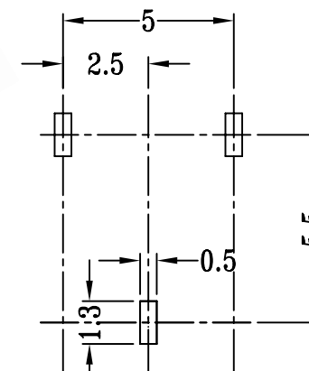
P.C.B LAYOUT
